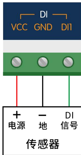
PNP/NPN接法
