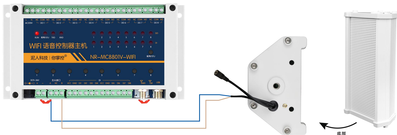
主机接语音音柱从机
