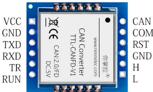
排针接口
