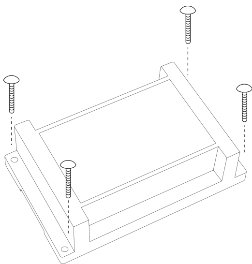
定位孔安装
