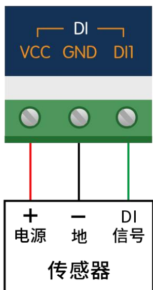
PNP/NPN接法
