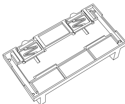
导轨安装
