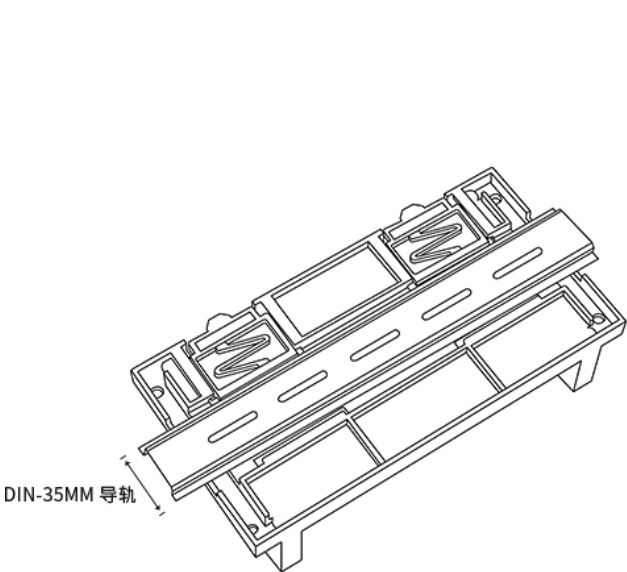
导轨安装
