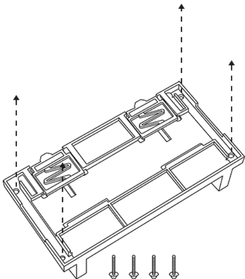
定位孔安装
