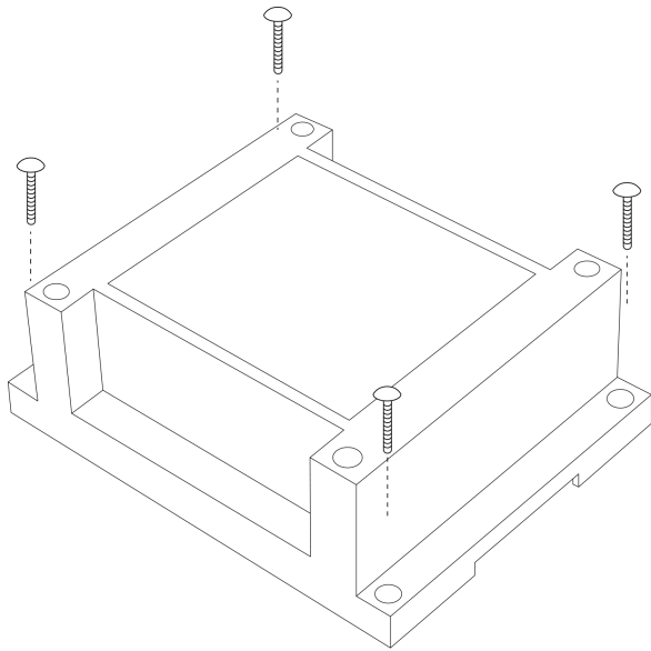
定位孔安装
