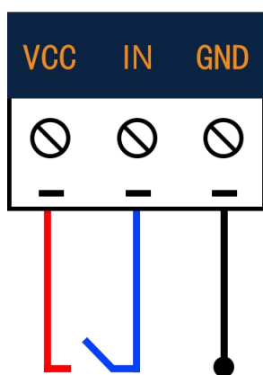
干触点接法
