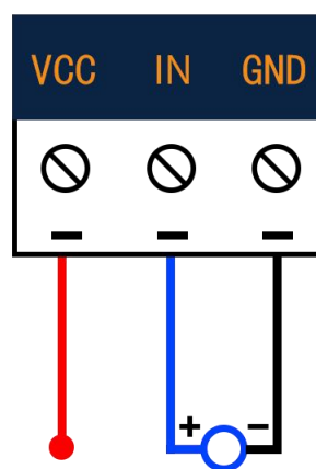
PNP湿触点接法
