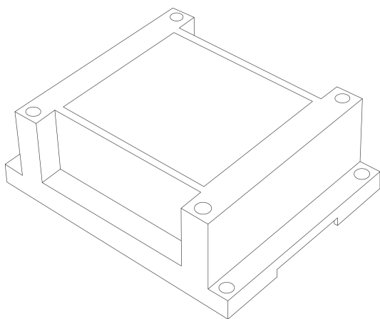
定位孔安装
